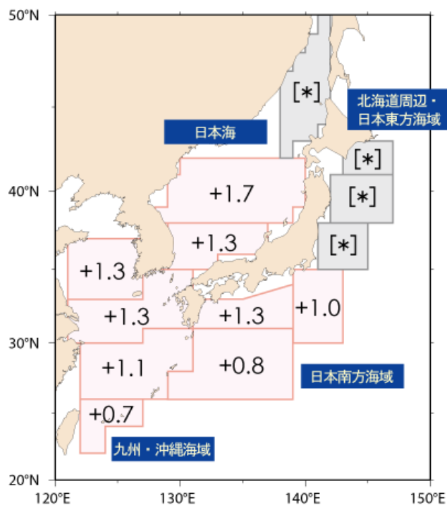
第2部 図2.2-1 日本近海の海域平均海面水温(年平均)の長期変化傾向(°C/100年) (正)
